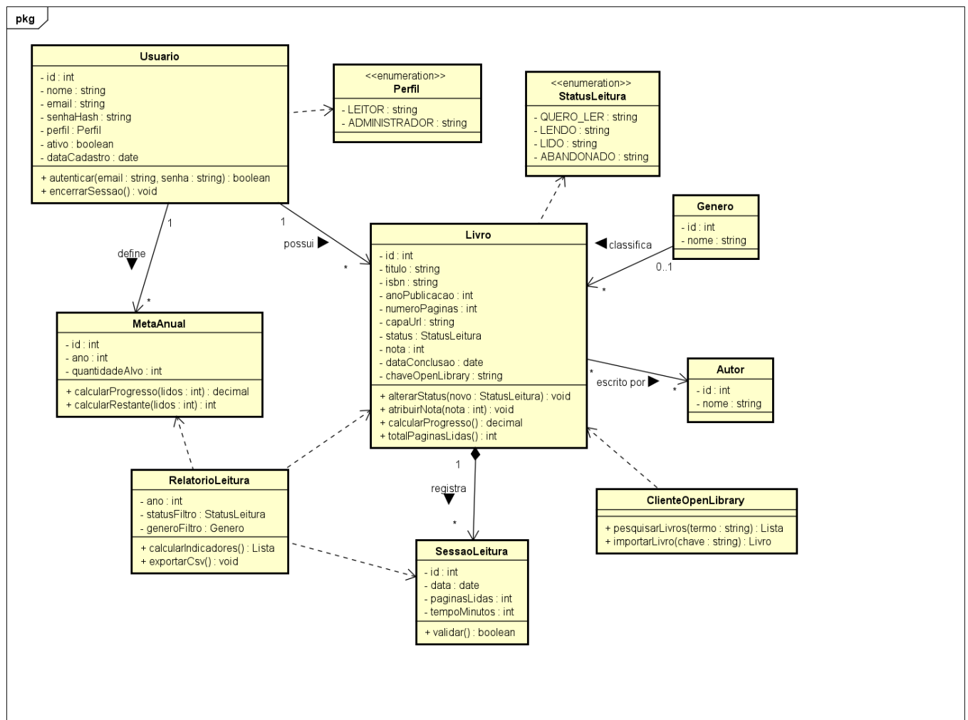
Figura 1 — Diagrama de classes (UML) do Estante.
