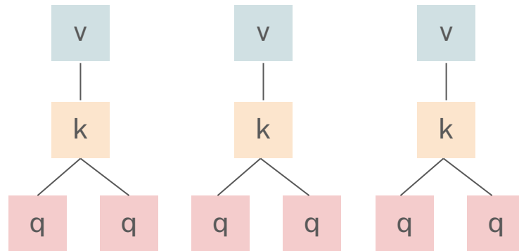
Grouped-query attention
