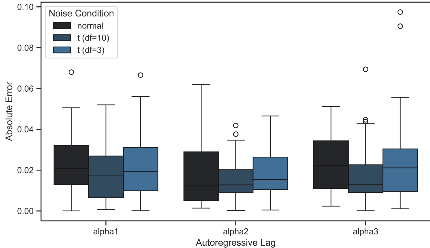
Distribution of Absolute Error for Autoregressive Parameters (K=13): ER
