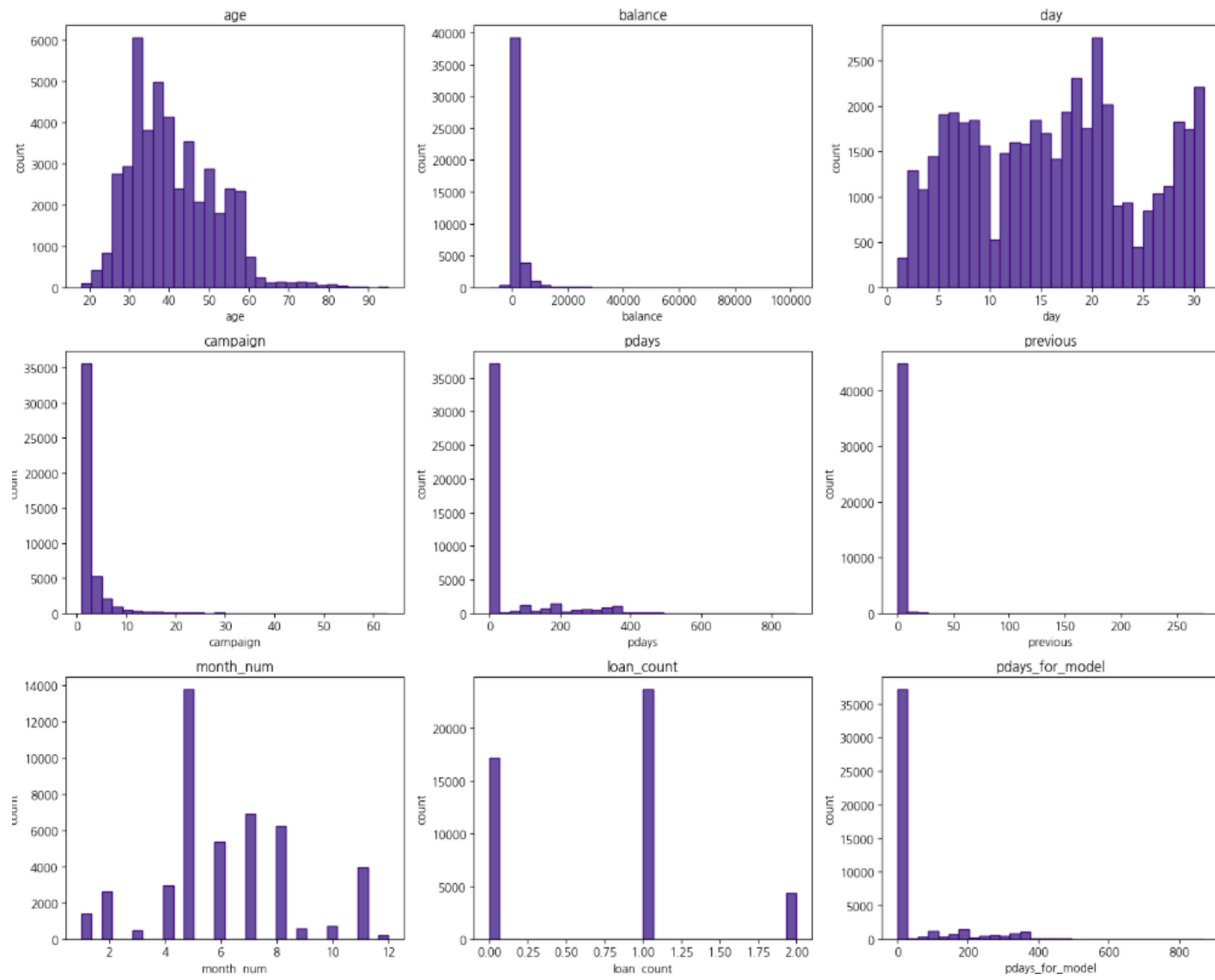
▲ 수치형 변수 분포
