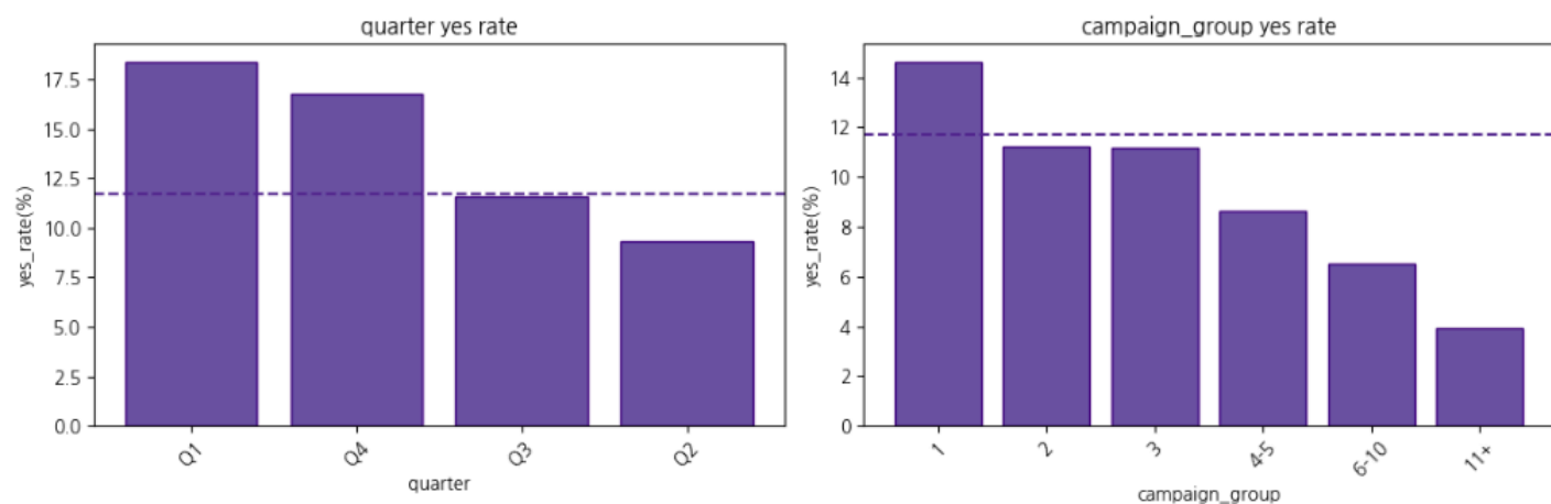
▲ 분기별 가입률, 현재 캠페인 연락 횟수 구간별 가입률
