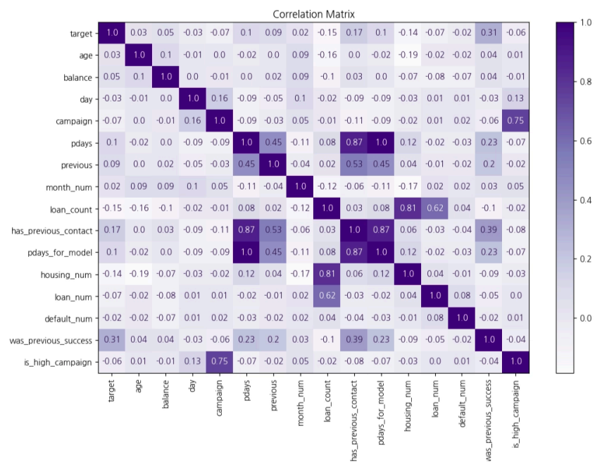
▲ 수치형 변수 상관관계 히트맵
