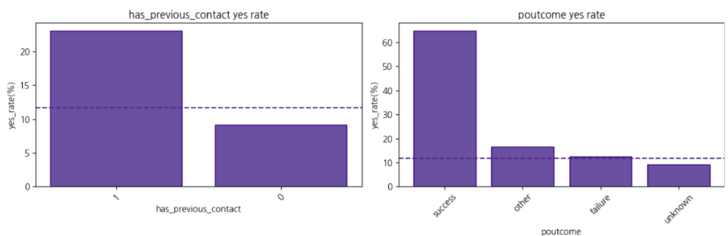
▲ 이전 연락 여부별 가입률, 이전 캠페인 결과별 가입률
