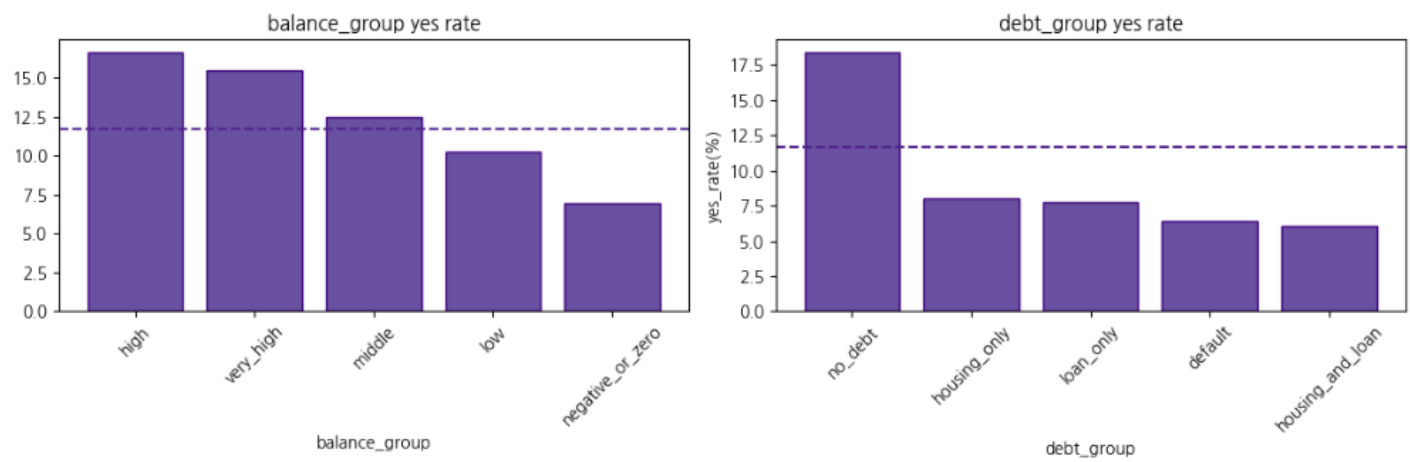
▲ 잔고 구간별 가입률, 금융 부담 그룹별 가입률
