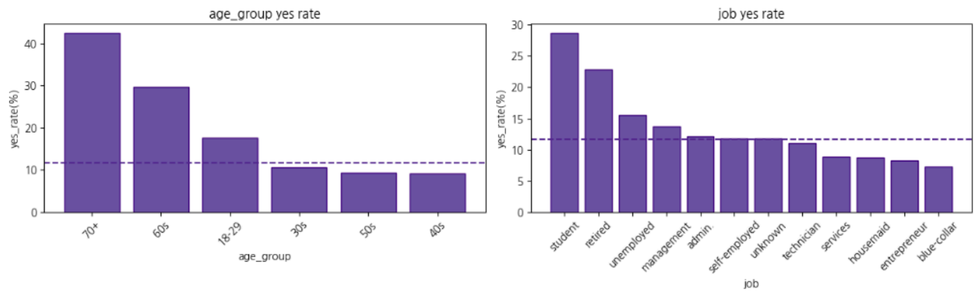
▲ 나이대별 가입률, 직업별 가입률
