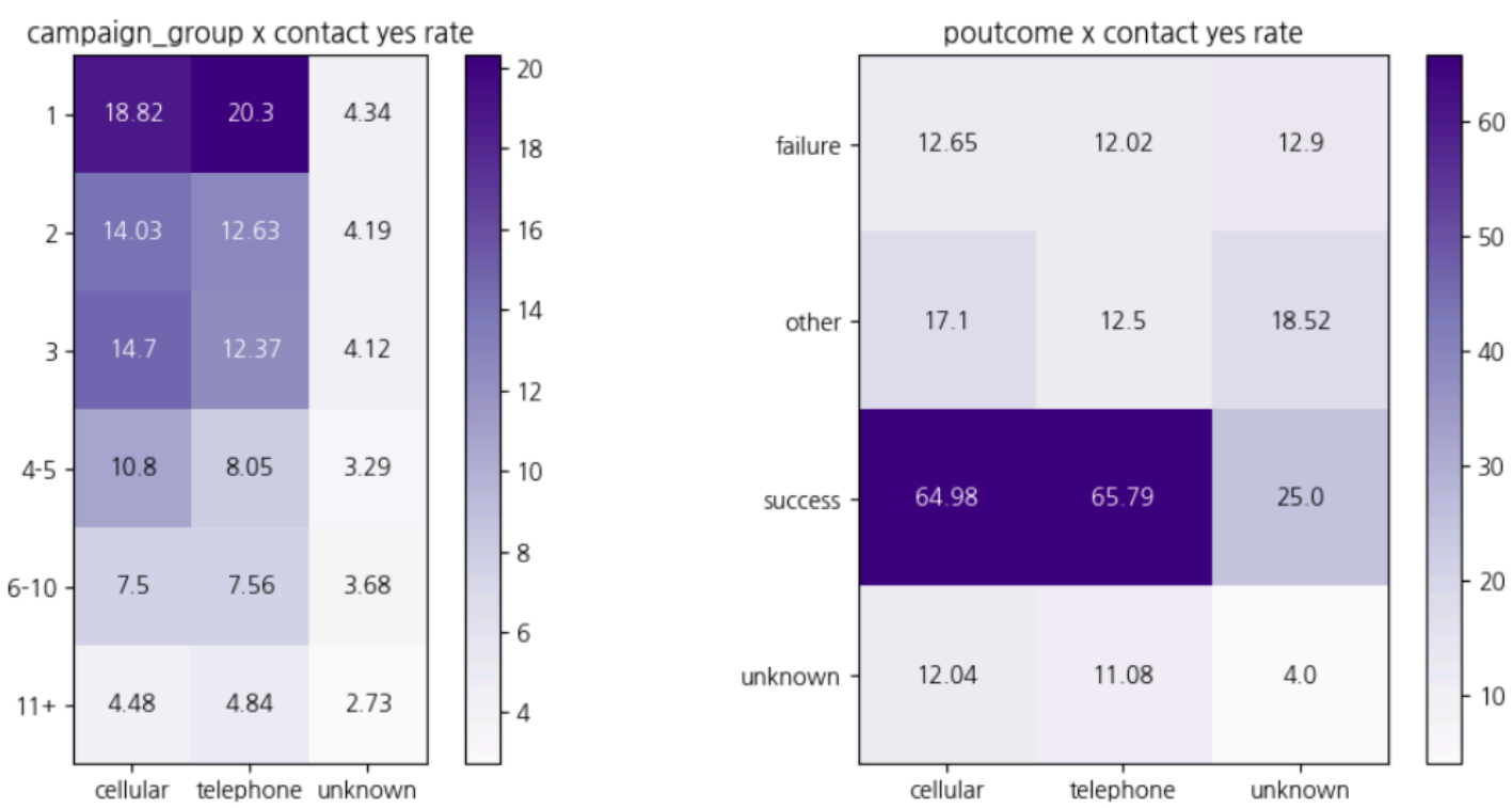
▲ 캠페인 구간 × 연락 수단 가입률, 이전 캠페인 결과 × 현재 연락 수단 가입률
