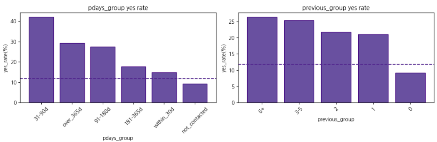
▲ 이전 연락 후 경과일 구간별 가입률, 이전 연락 횟수 구간별 가입률
