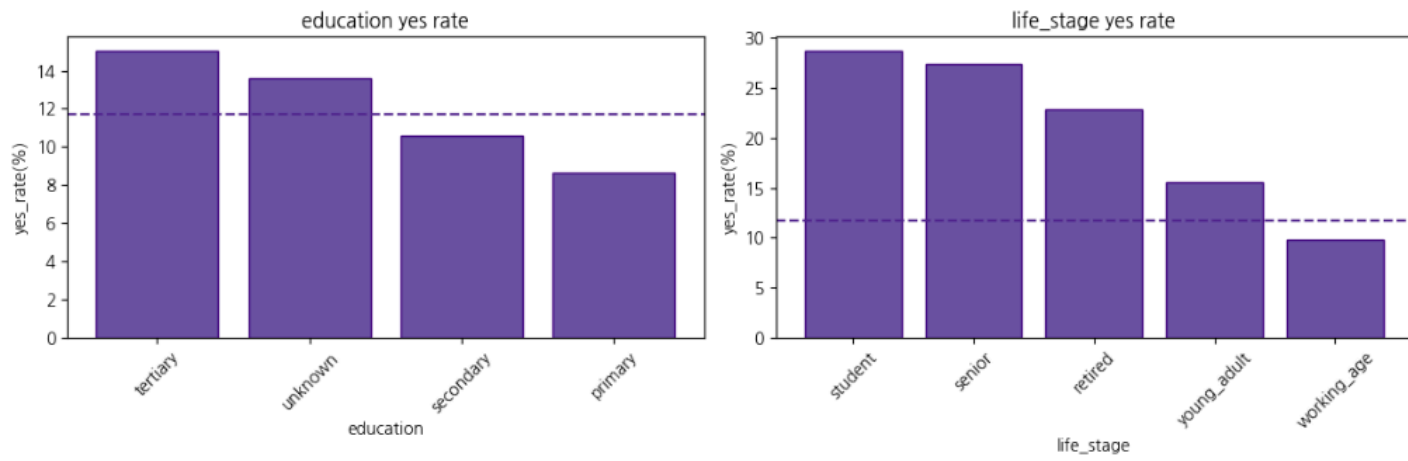
▲ 교육 수준별 가입률, 생애단계별 가입률
