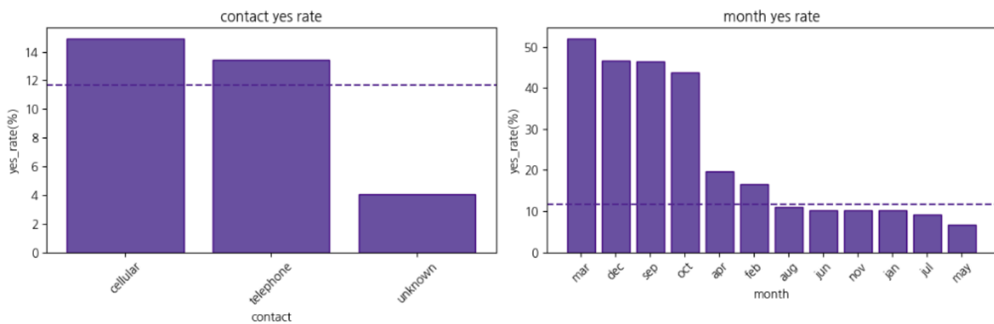
▲ 연락 수단별 가입률, 연락 월별 가입률
