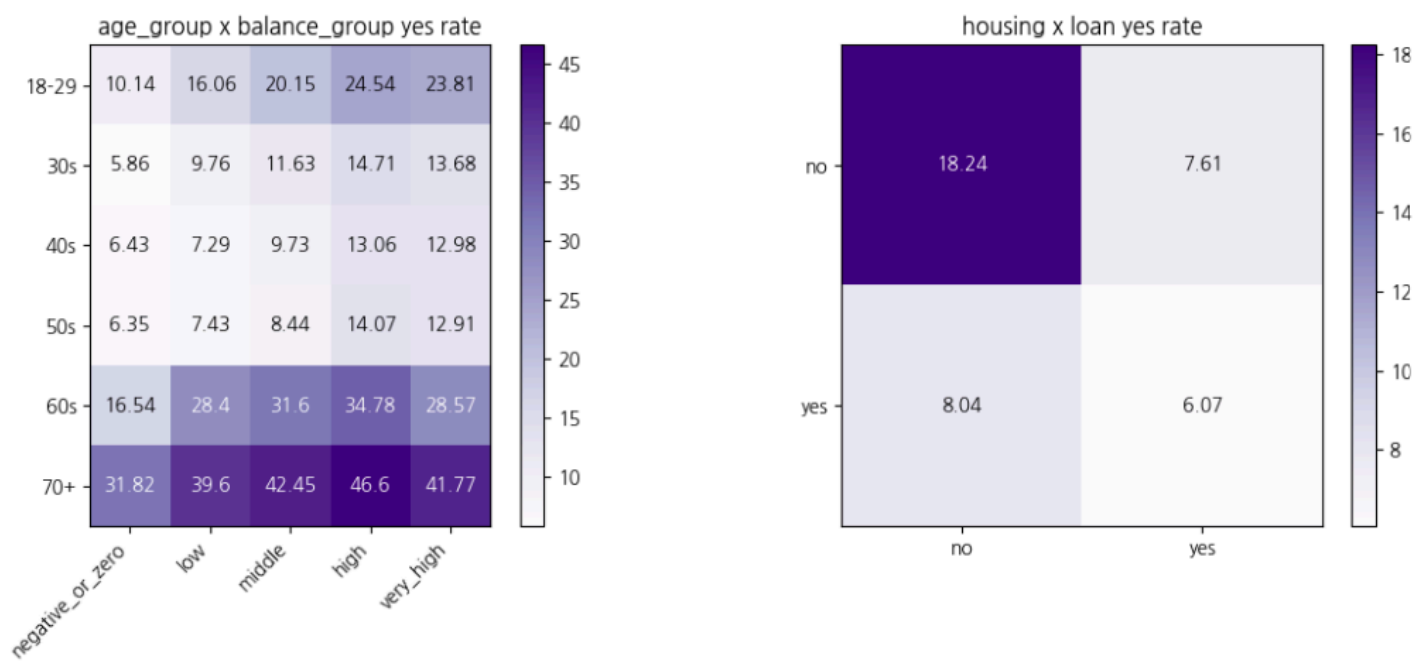
▲ 나이대 × 잔고 구간 가입률, 주택담보대출 × 개인대출 가입률
