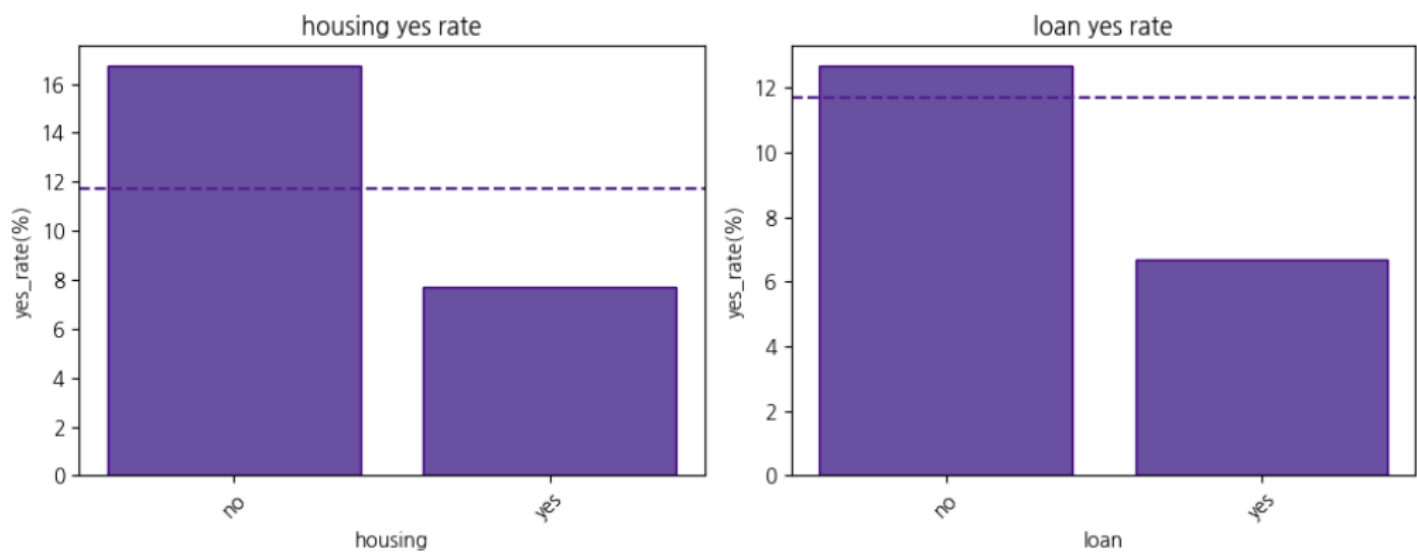
▲ 주택담보대출 여부별 가입률, 개인대출 여부별 가입률
