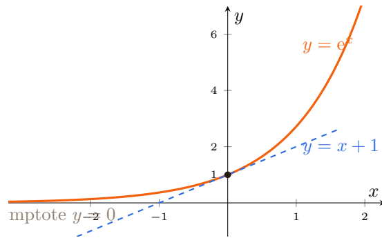
Figure 2 — Courbe de \exp : convexe, asymptote y = 0 en -\infty , au-dessus de sa tangente y = x + 1 .
