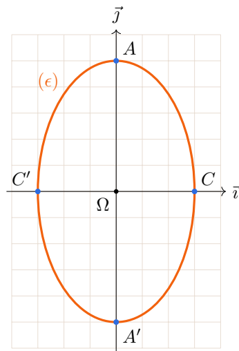
Ellipse (\epsilon) de centre \Omega(1; -2) , sommets A, A', C, C' .
