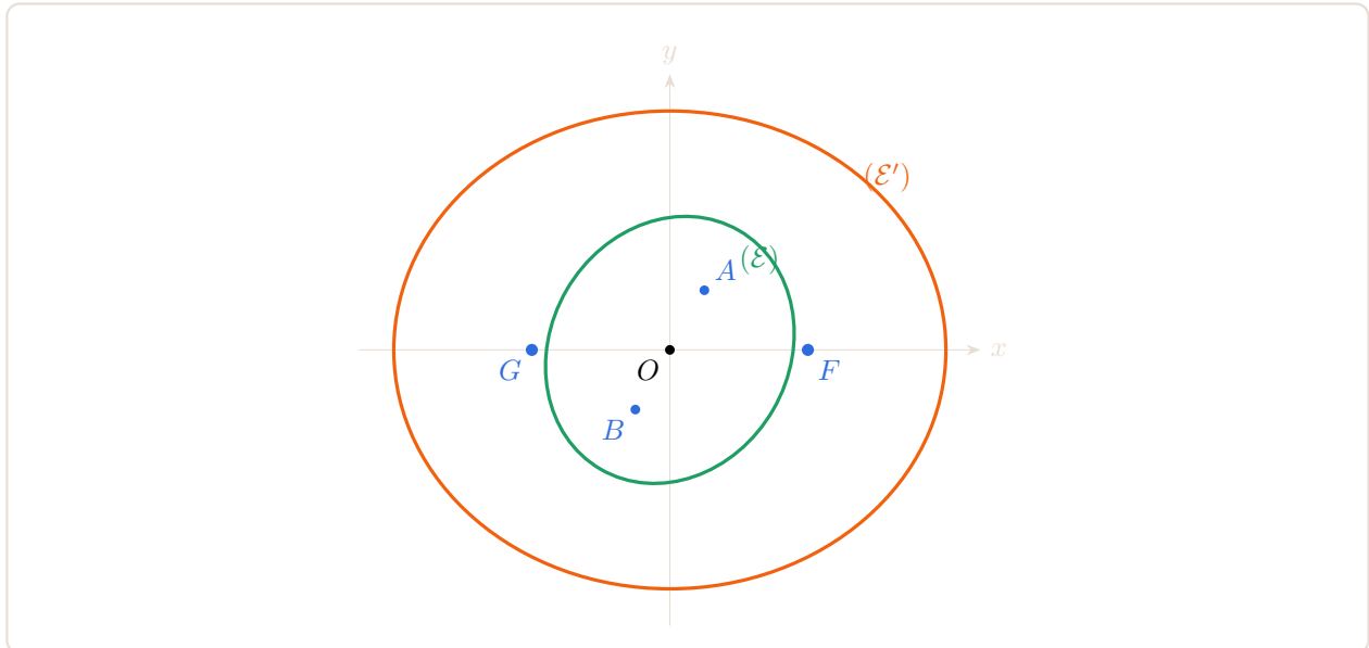
(\mathcal{E}') en orange (foyers F, G ) et son image (\mathcal{E}) en vert (foyers A, B ).
