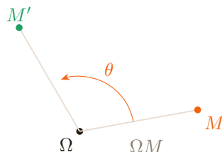
Figure 2 — Action d'une rotation de centre \Omega et d'angle \theta .
