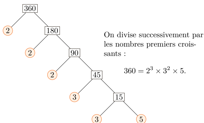
Figure 1.5 — Arbre de décomposition de 360 en facteurs premiers.
