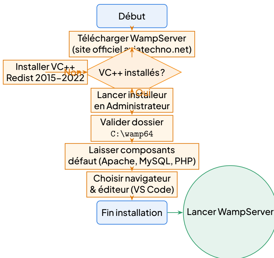
Organigramme des étapes d'installation de WampServer avec vérification des prérequis VC++
