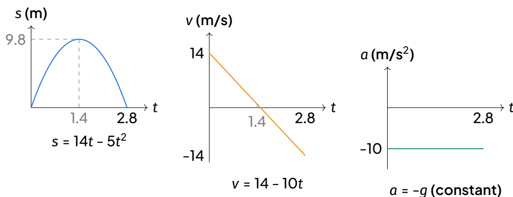
Graphiques déplacement-temps, vitesse-temps et accélération-temps pour la balle lancée vers le haut à 14 \text{ m s}^{-1} .
