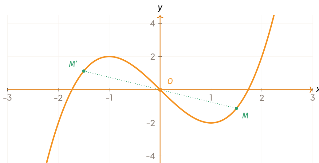
Courbe de f(x) = x^3 - 3x : l'origine O est centre de symétrie. Les points M(1,5; -1,125) et M'(-1,5; 1,125) sont échangés par la symétrie de centre O .
