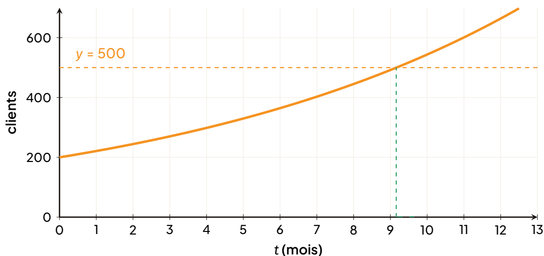
Courbe de N(t) = 200 e^{0,1t} et lecture graphique du seuil de 500 clients.
