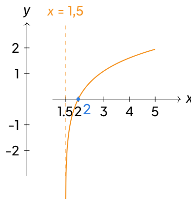
Courbe de f(x) = \ln(2x - 3) .
