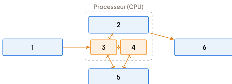
Schéma fonctionnel de l'ordinateur à compléter (étiquettes 1 à 6).
