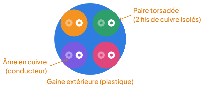
Coupe transversale d'un câble à paires torsadées : 4 paires de fils de cuivre enfermées dans une gaine plastique.
