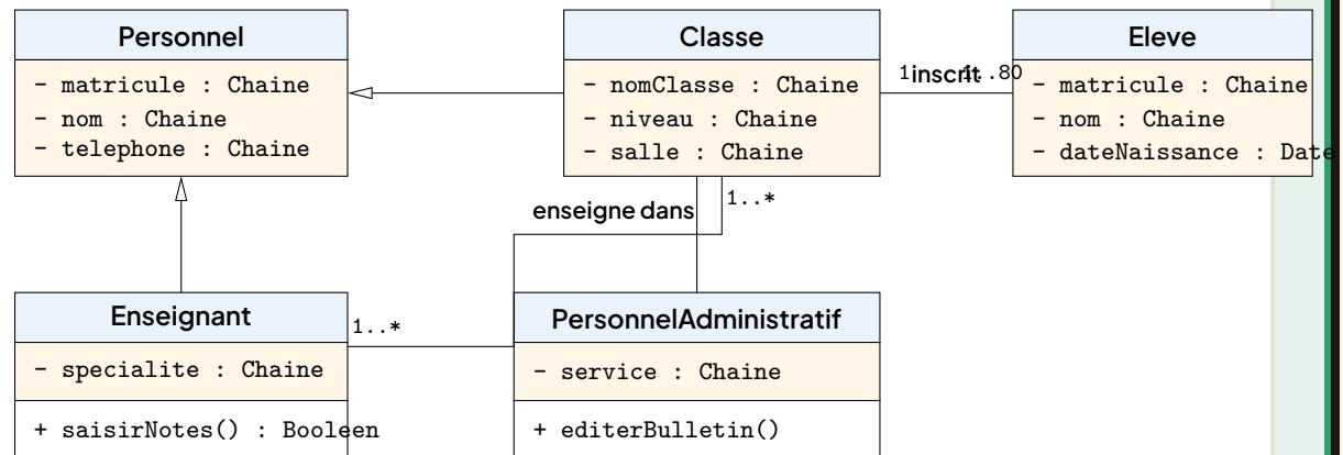
Diagramme de classes du lycée : héritage (triangles vides vers Personnel ) et associations.
