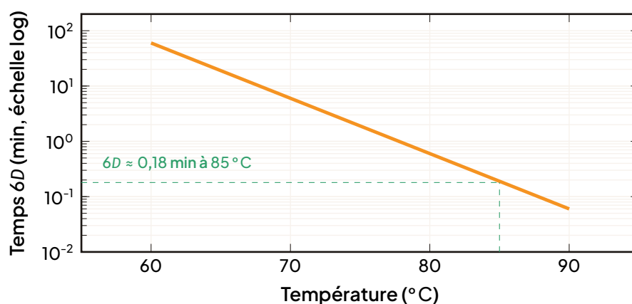
Courbe du temps de réduction 6D en fonction de la température (échelle semi-logarithmique). Lecture graphique à 85 °C : 6D \approx 0,18 min.
