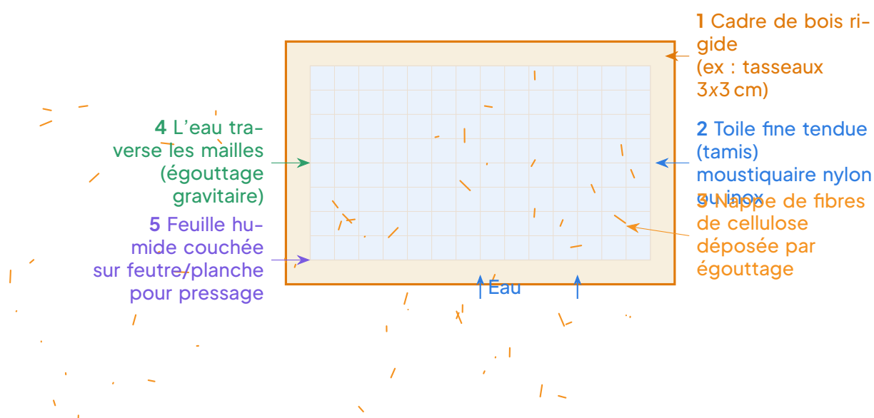
Schéma de principe du cadre à tamis (moule à papier) pour fabrication artisanale. 1 Cadre bois; 2 Toile (tamis); 3 Fibres retenues formant la feuille; 4 Égouttage de l'eau; 5 Couchage (transfert de la feuille humide sur support absorbant) avant pressage.
