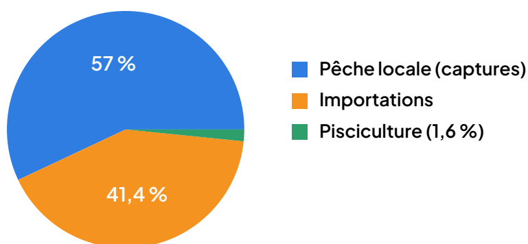
Diagramme circulaire : structure de l'approvisionnement en poisson au Cameroun (estimation). Les importations représentent près de 42 % de l'offre.
