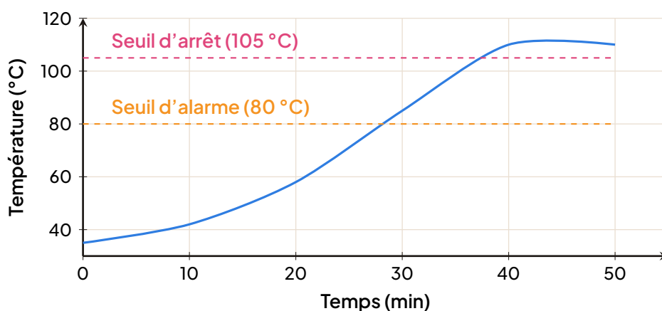
Figure 1 : évolution de la température du palier côté entraînement avant l'arrêt d'urgence. Source : système SCADA, station de Nkolfoulou, 15/03/2026.
