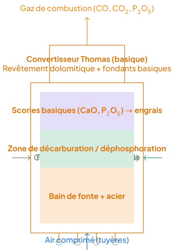
Figure 2 – Schéma du convertisseur Thomas (1878). L'air comprimé traverse la fonte phosphoreuse; le phosphore passe dans les scories basiques (engrais), l'acier est produit en 15–20 min à bas coût. Rails, coques de navires, canons deviennent abordables.
