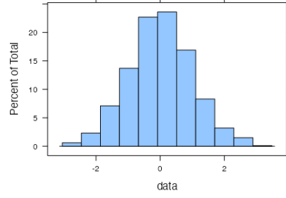
(d) A histogram plot.
