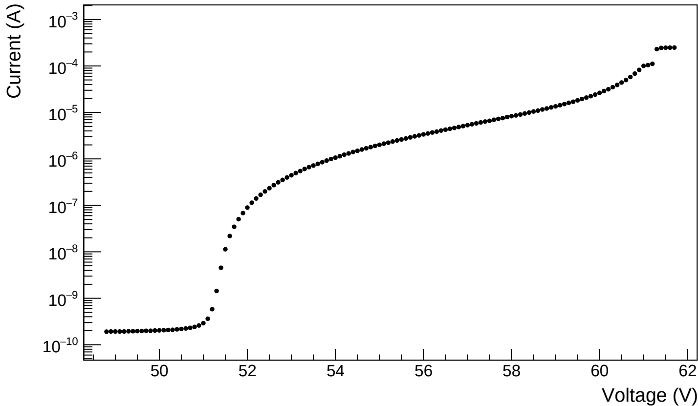
Sensor A1 - 125 °C, 5 h - T = 21 °C
