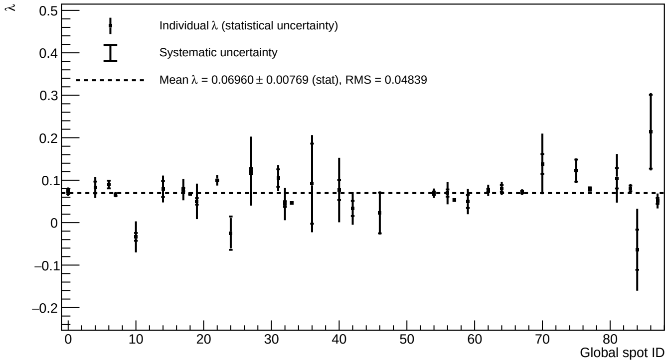
A1_v=5_annealing_T=125_h=25 - Exponential fit parameter \lambda - annealing_T=125_h=25
