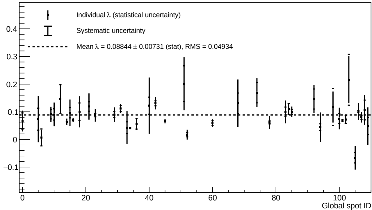
B1_v=3_annealing_T=125_h=25 - Exponential fit parameter \lambda - annealing_T=125_h=25
