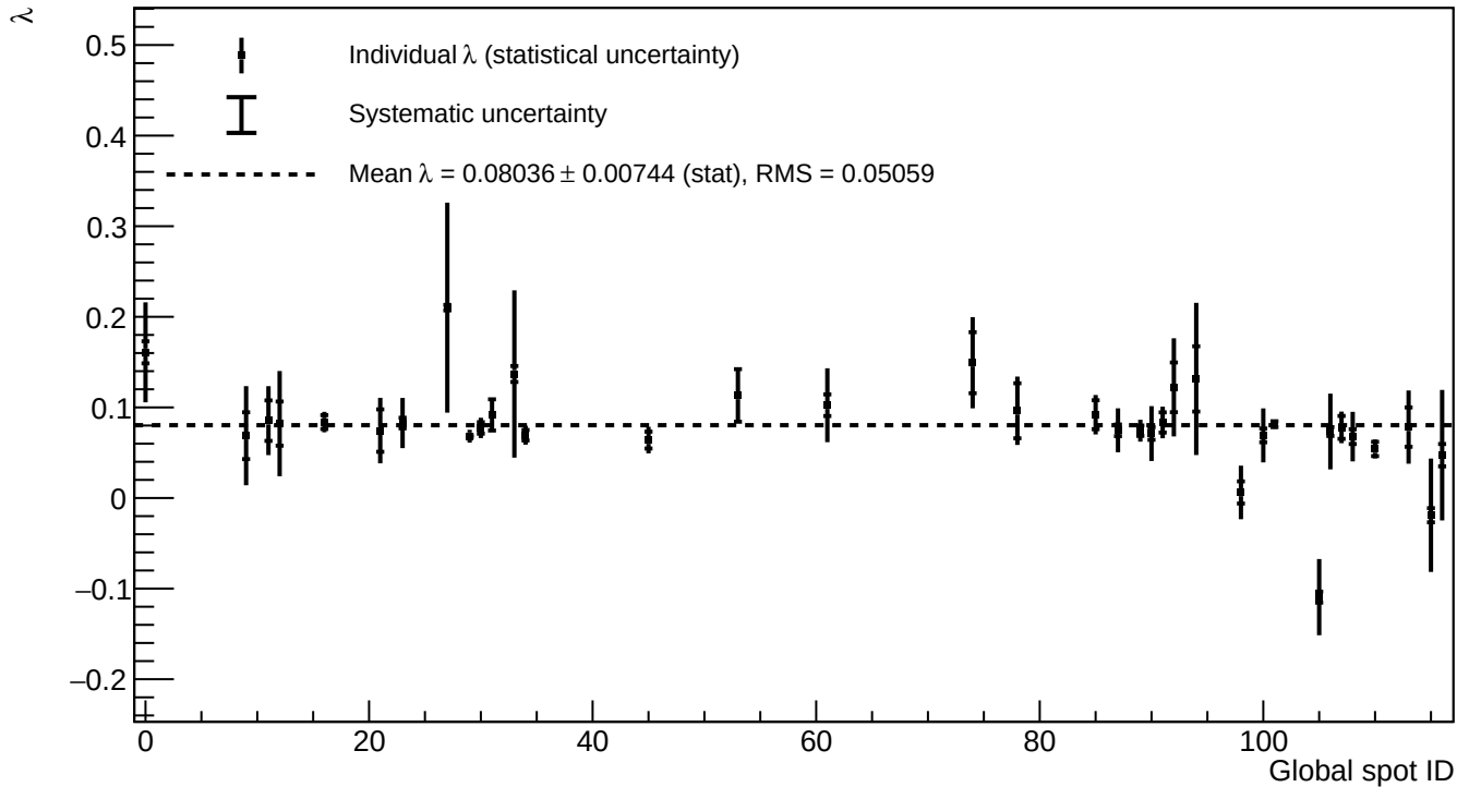
B1_v=3_annealing_T=150_h=5 - Exponential fit parameter \lambda - annealing_T=150_h=5
