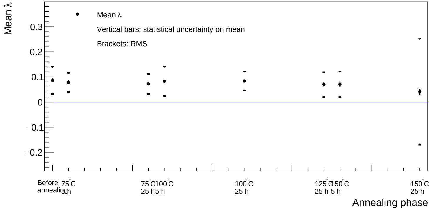
Sensor A1 - Mean fit parameter \lambda vs annealing phases
