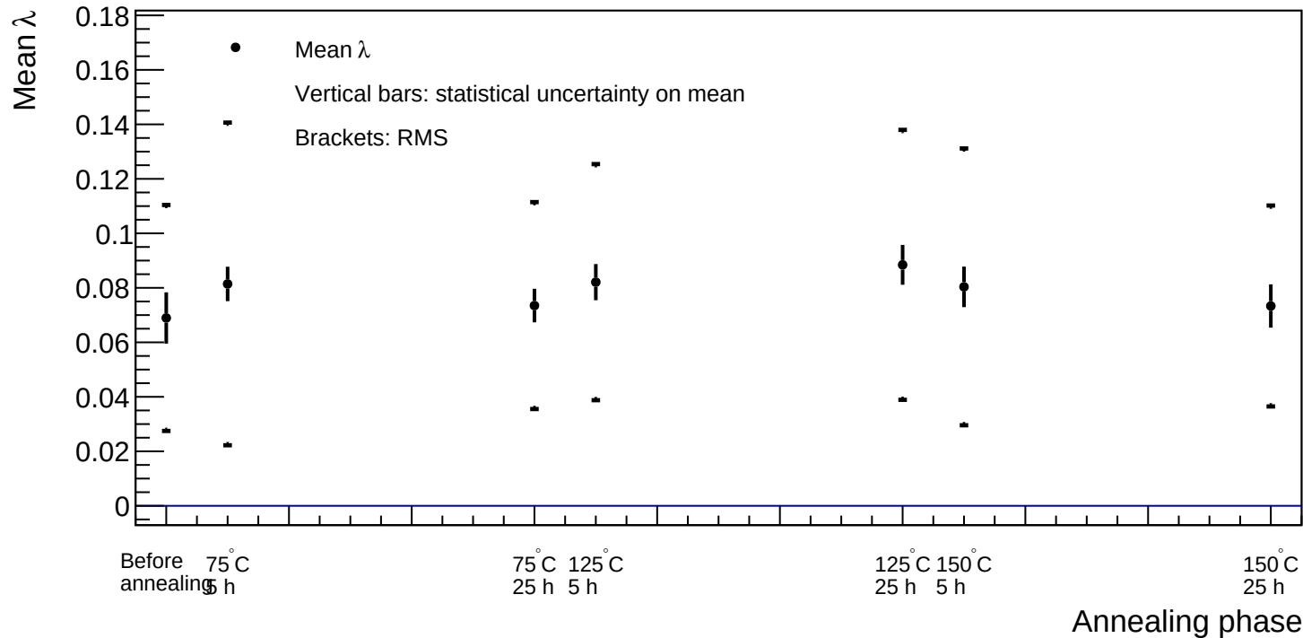
Sensor B1 - Mean fit parameter \lambda vs annealing phases
