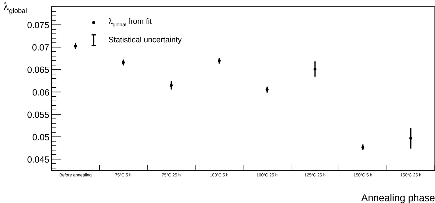
Sensor A1 - Simultaneous fit parameter \lambda vs annealing phases
