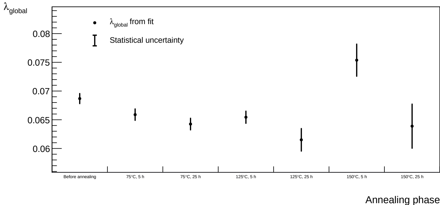
Sensor B1 - Simultaneous fit parameter \lambda vs annealing phases
