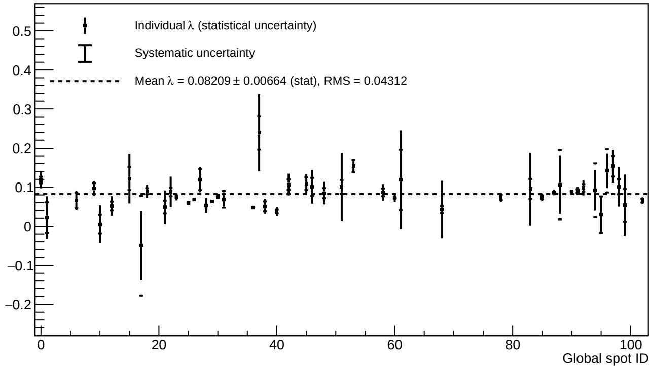
B1_v=3_annealing_T=125_h=5 - Exponential fit parameter \lambda - annealing_T=125_h=5
