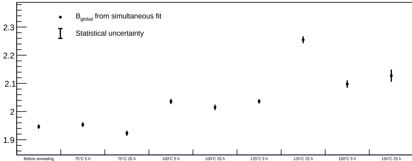
Sensor B1 - Simultaneous fit parameter B vs annealing phases
