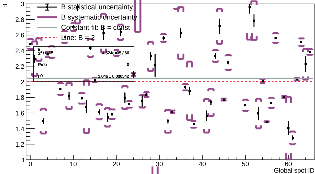
Sensor A1 - Power-law exponent B - annealing T=75_h=5
