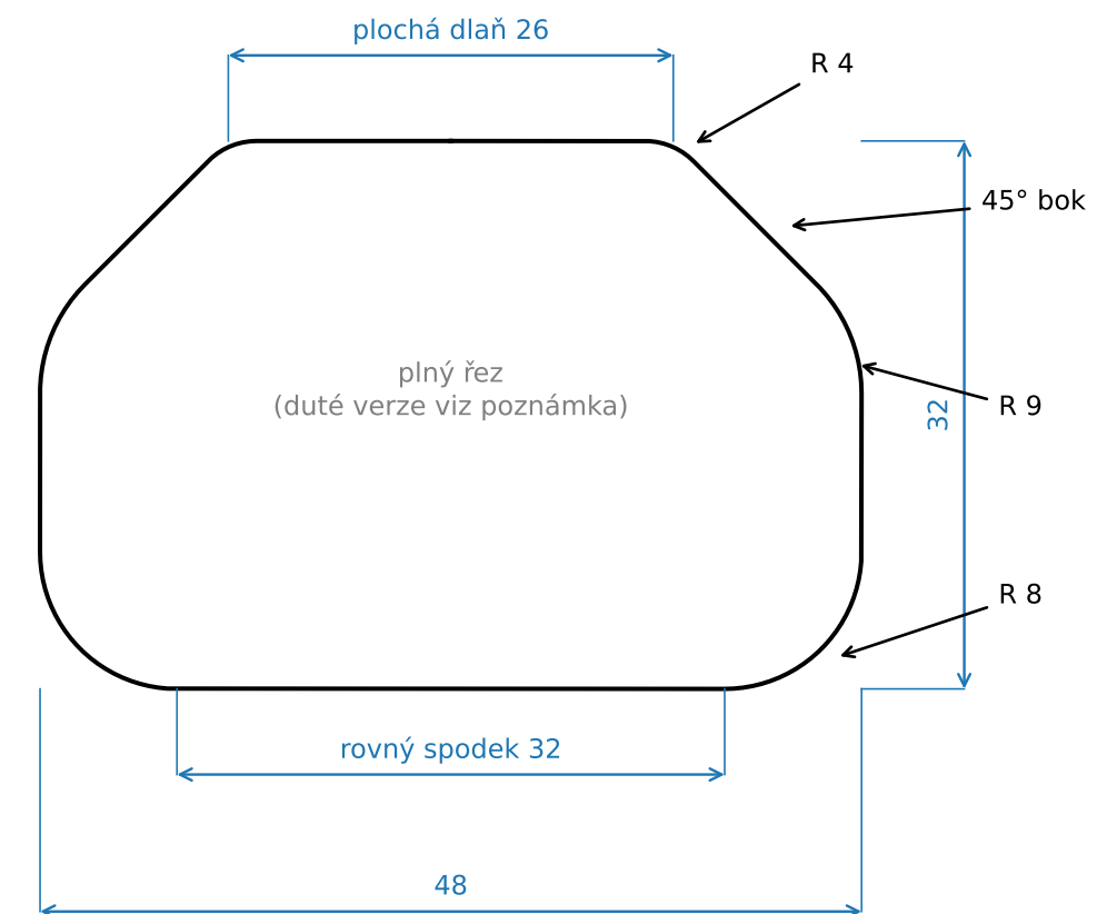
Příčný řez tyčí mimo trn (dlaň nahoře)
