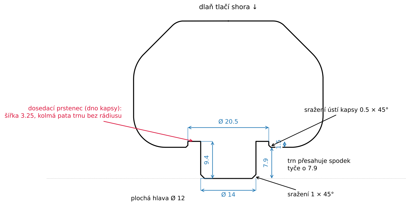
Řez A-A osou trnu (pracovní orientace: trn dole)
