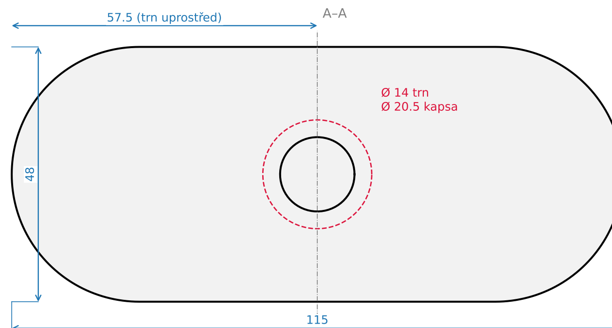
Pohled shora na tyč (trn leží mezi prostředníčkem a prsteníčkem)
