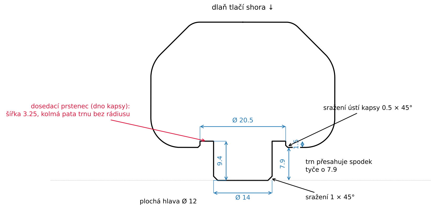
Řez A-A osou trnu (pracovní orientace: trn dole)
