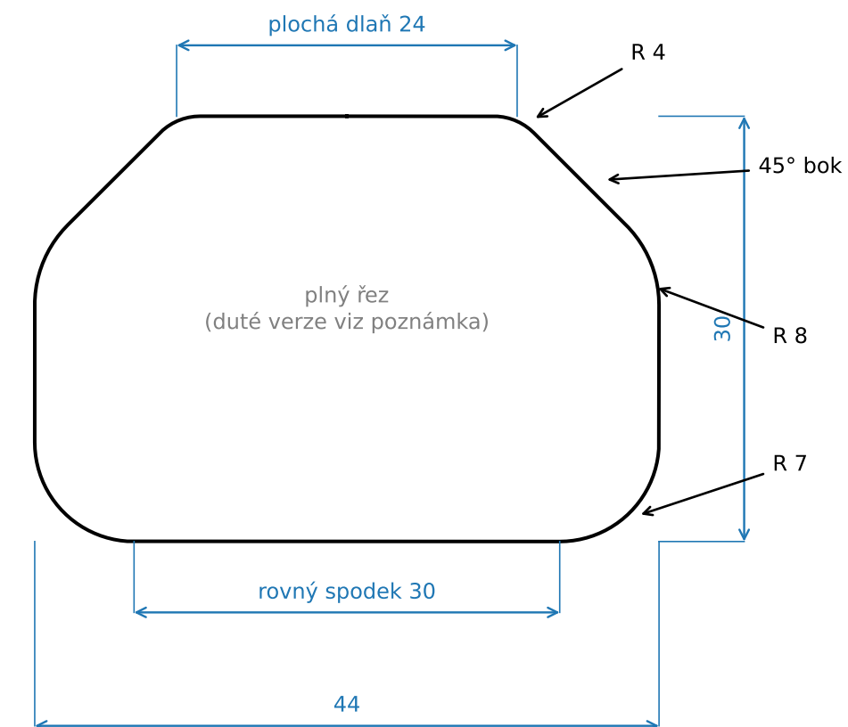
Příčný řez tyčí mimo trn (dlaň nahoře)
