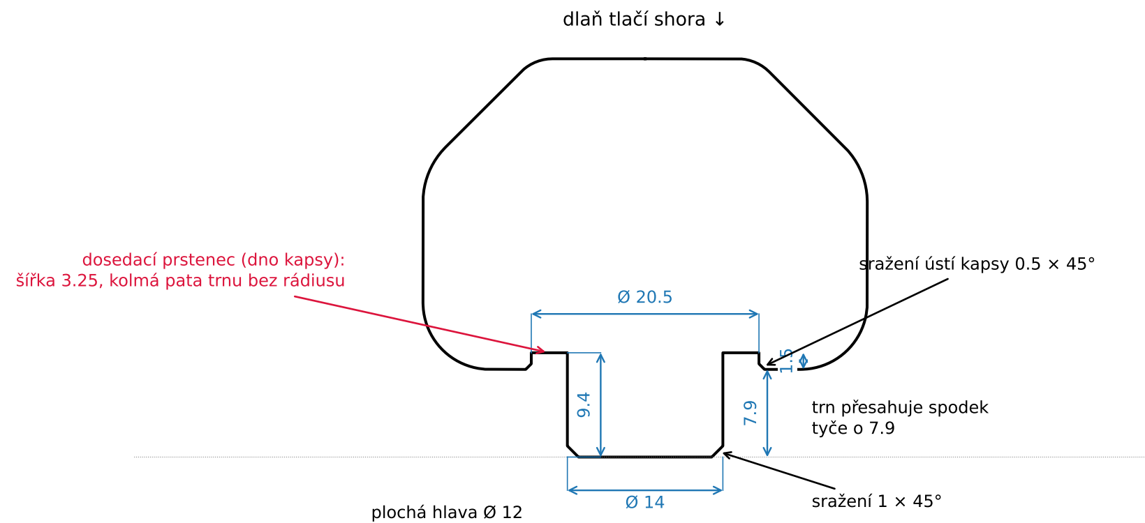
Řez A-A osou trnu (pracovní orientace: trn dole)
