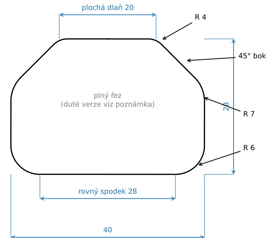
Příčný řez tyčí mimo trn (dlaň nahoře)
