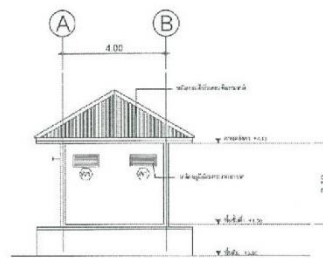
รูปด้านที่ 2 SCALE 1:100
