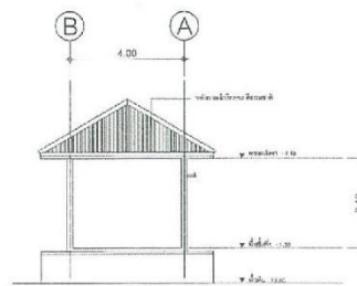
รูปด้านที่ 4 SCALE 1:10
