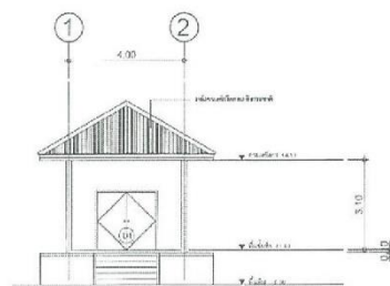
รูปด้านที่ 1 SCALE 1:100
