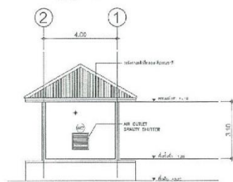
รูปด้านที่ ๓ SCALE 1:100
