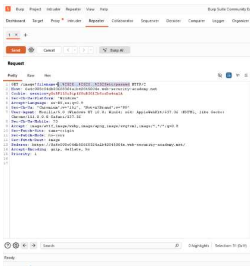
Figura 6. Petición modificada en Repeater con el payload doblemente codificado ../../etc/passwd.
