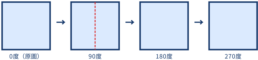
正方形旋轉對稱：每轉90度重疊一次（4重）
