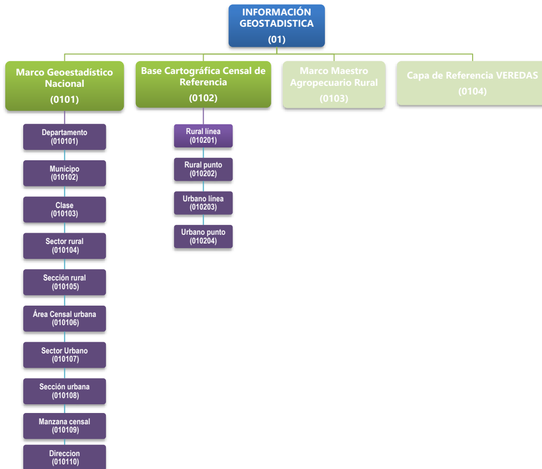
Ilustración 2 Representación Tema Información Geoestadística MGN.
