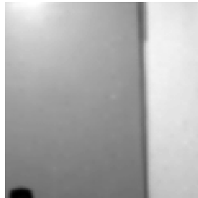
epit
