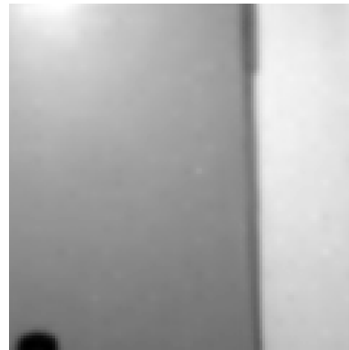
det
