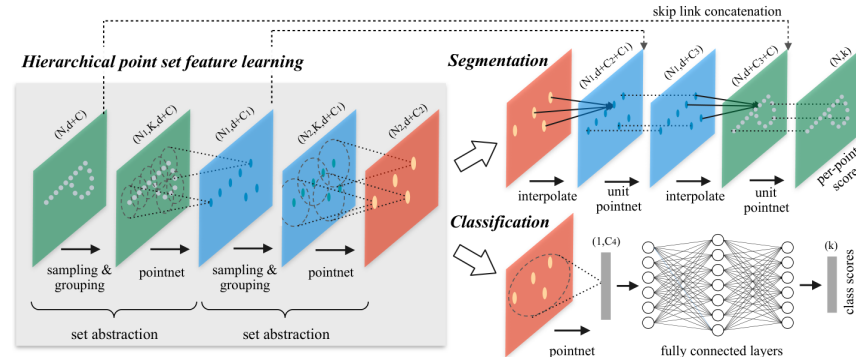
Abbildung 5: Architektur von PointNet++ mit hierarchischen Set-Abstraktions-Stufen sowie Segmentierungs- und Klassifikationszweig [24].
