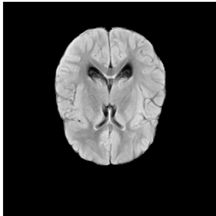
Ours (Ensemble)
