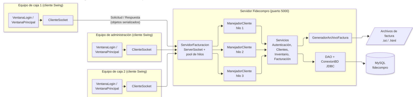
Arquitectura general de la solución
