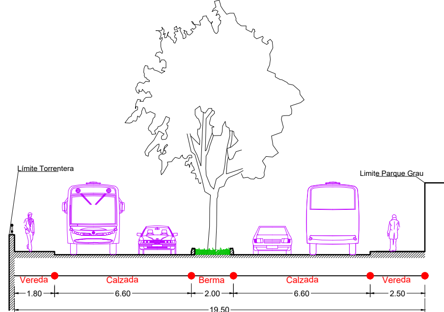
SECCIÓN VÍAL 6-6: ANILLO VIAL AV. LA MARINA TRAMO PUENTE GRAU
