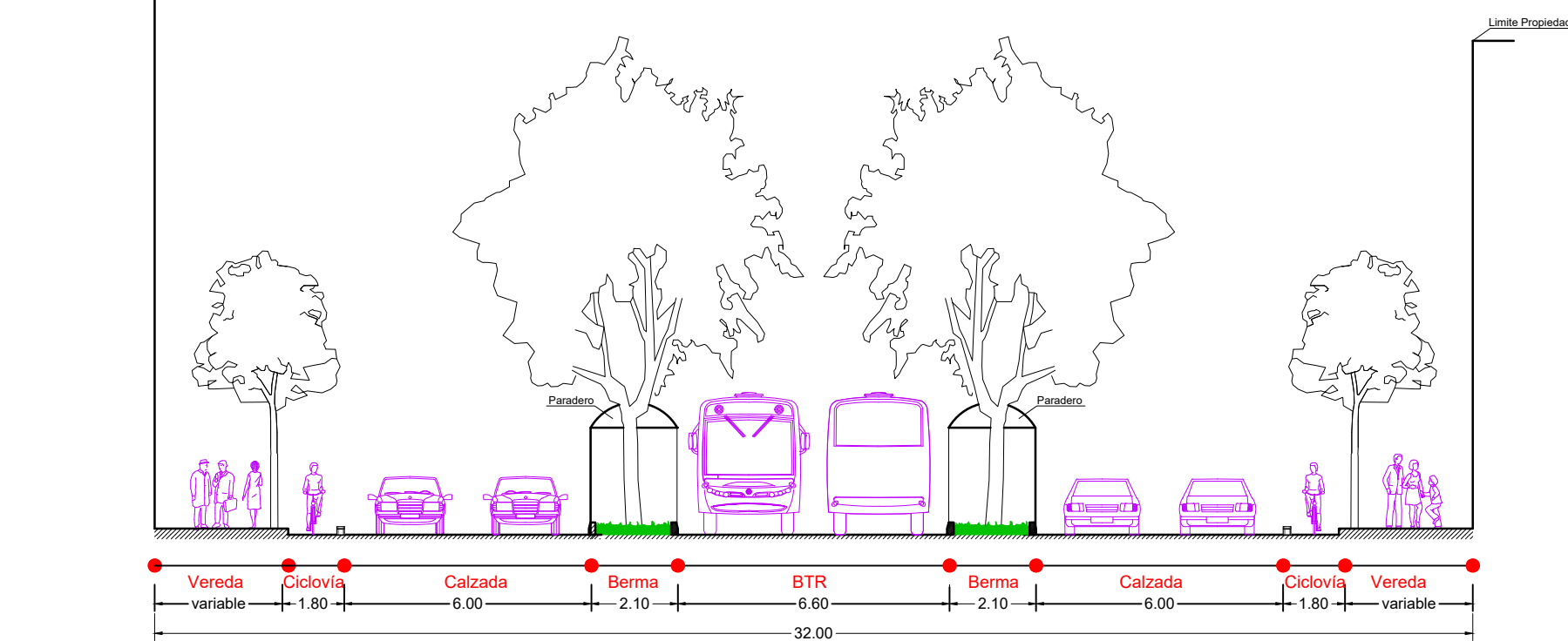
SECCIÓN VÍAL 3-3: VIA ARTERIAL AV. PARRA
