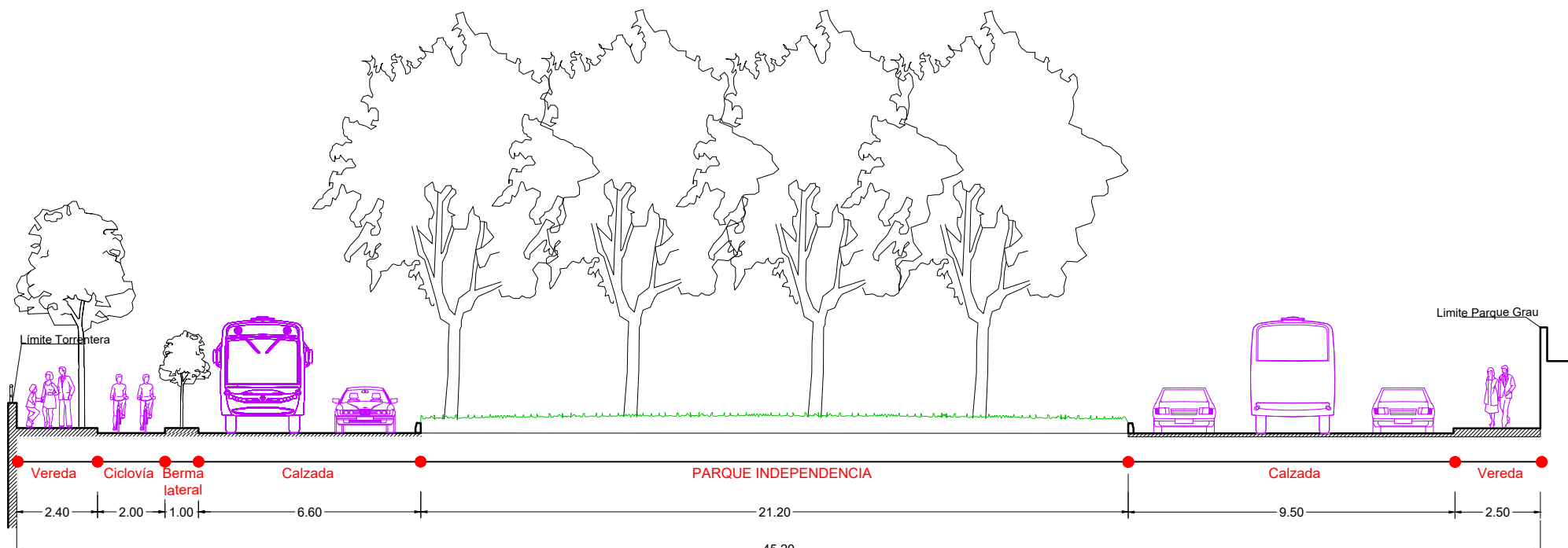
SECCIÓN VÍAL 6-6: ANILLO VIAL AV. LA MARINA TRAMO PUENTE GRAU
