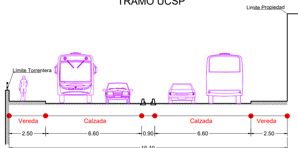
SECCIÓN VÍAL 4-4: ANILLO VIAL AV. JUAN DE LA TORRE TRAMO UCSP
