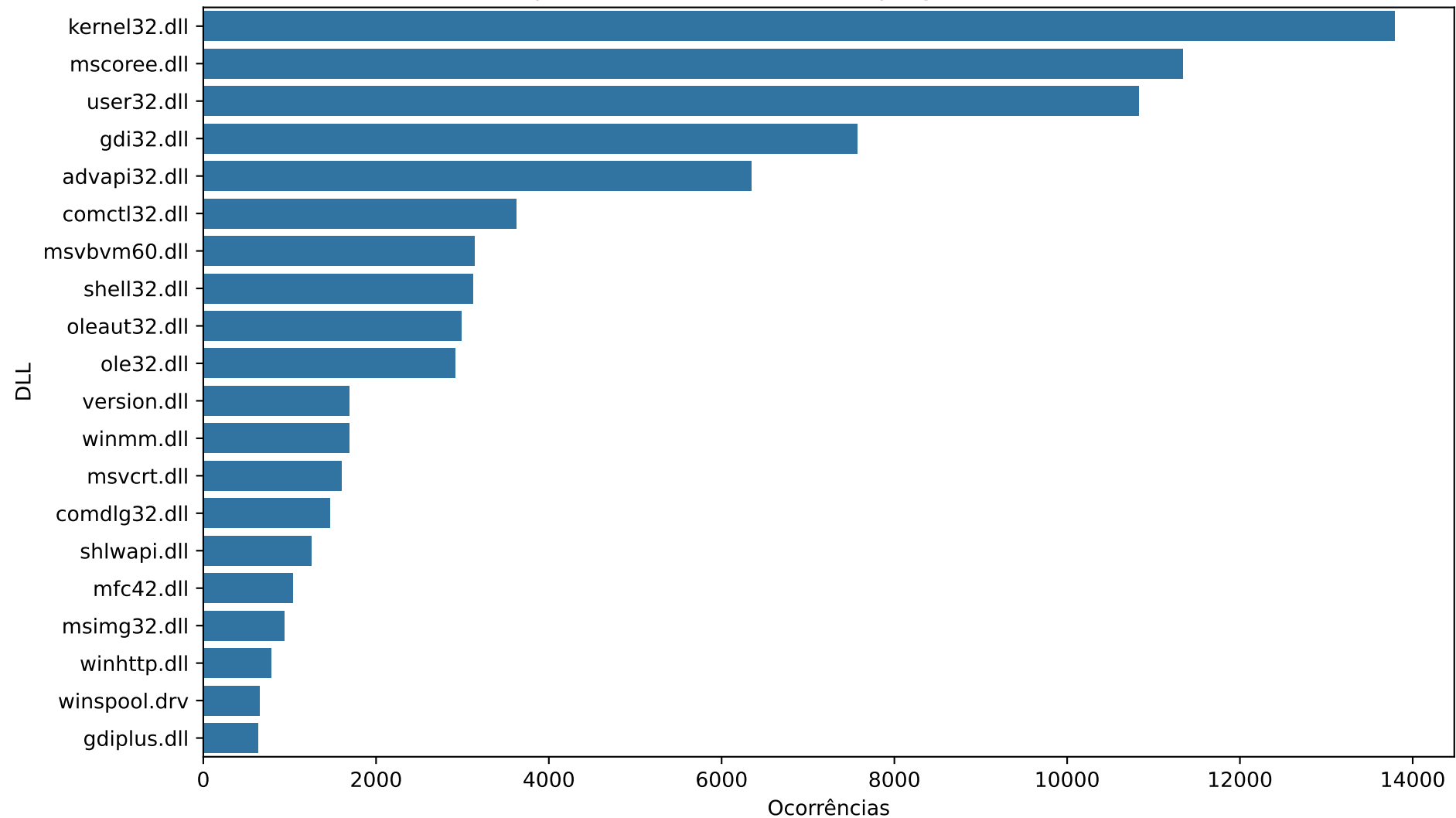
Top 20 DLLs mais usadas nos programas maliciosos
