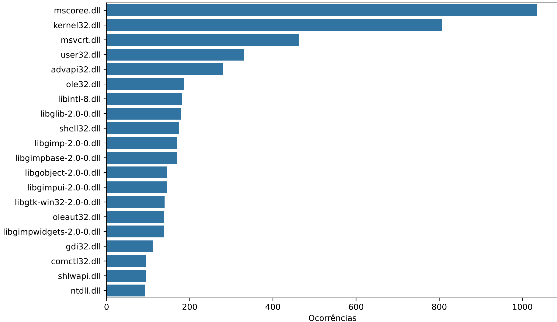
Top 20 DLLs mais usadas nos programas benignos
