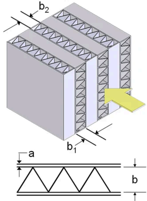
Plate-fin
