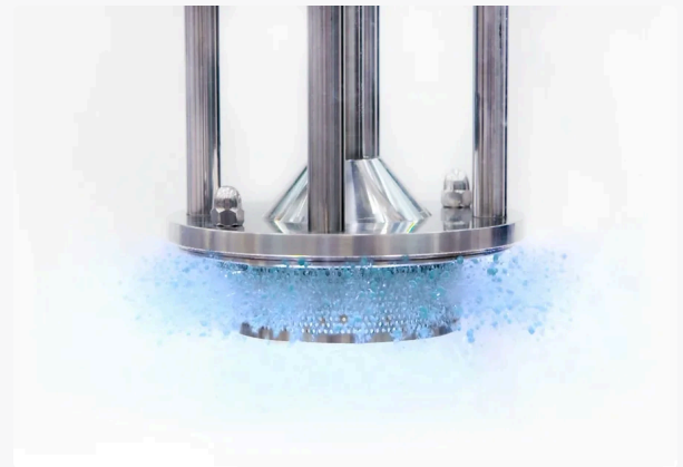
Dispersor rotor-estátor: cizalla localizada que rompe gotas. La P/V en esa zona supera 10-100× la del tanque agitado convencional.
