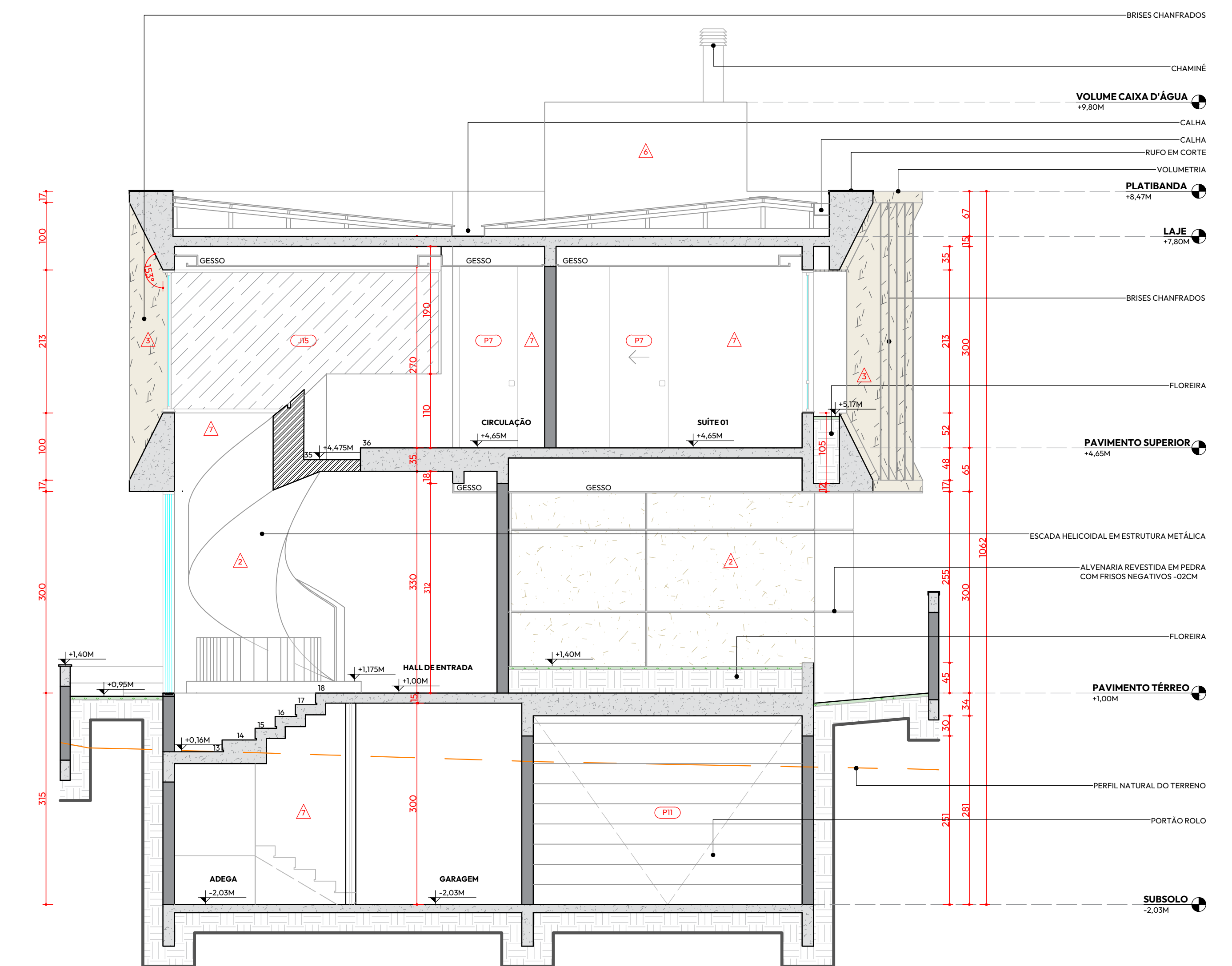
07 CORTE A/A ESCALA: 1/50
