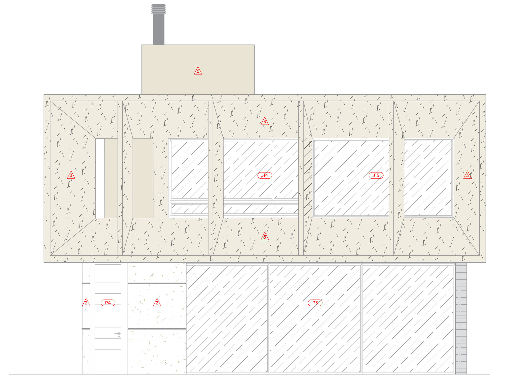
14 FACHADA POSTERIOR - E.03 ESCALA: 1/50
