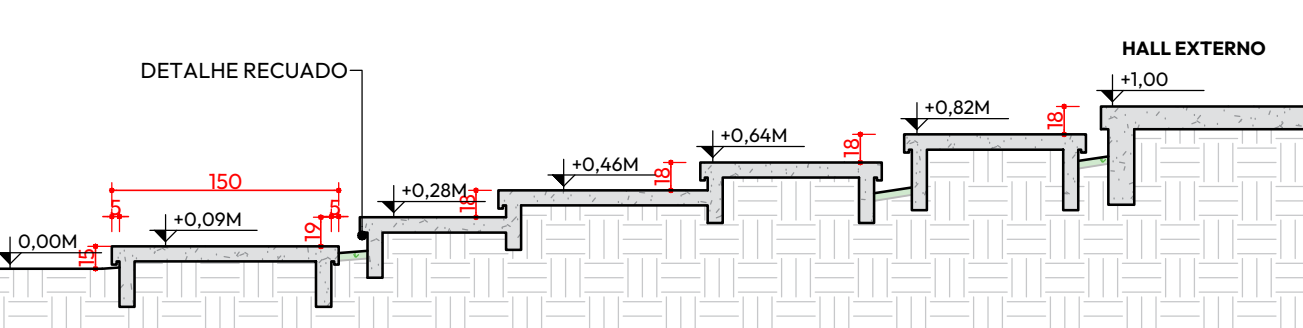
06 DET. EM CORTE DORMENTES ENTRADA ESCALA: 1/50
