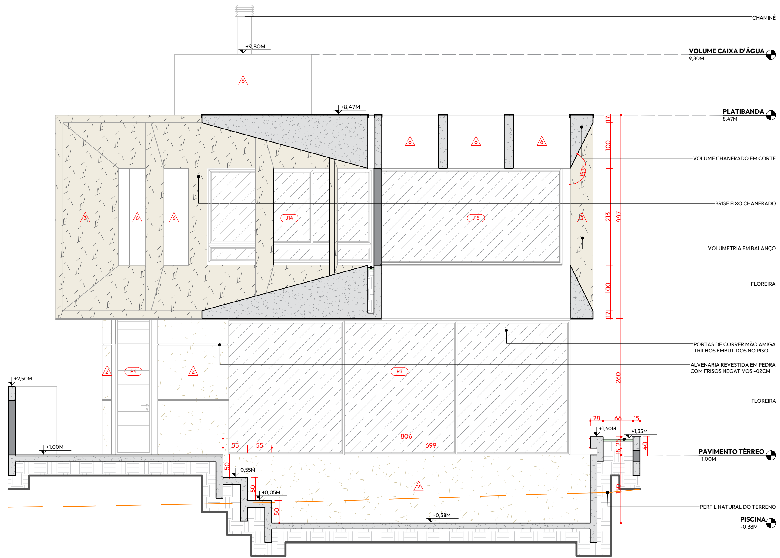
09 CORTE C/C ESCALA: 1/50
