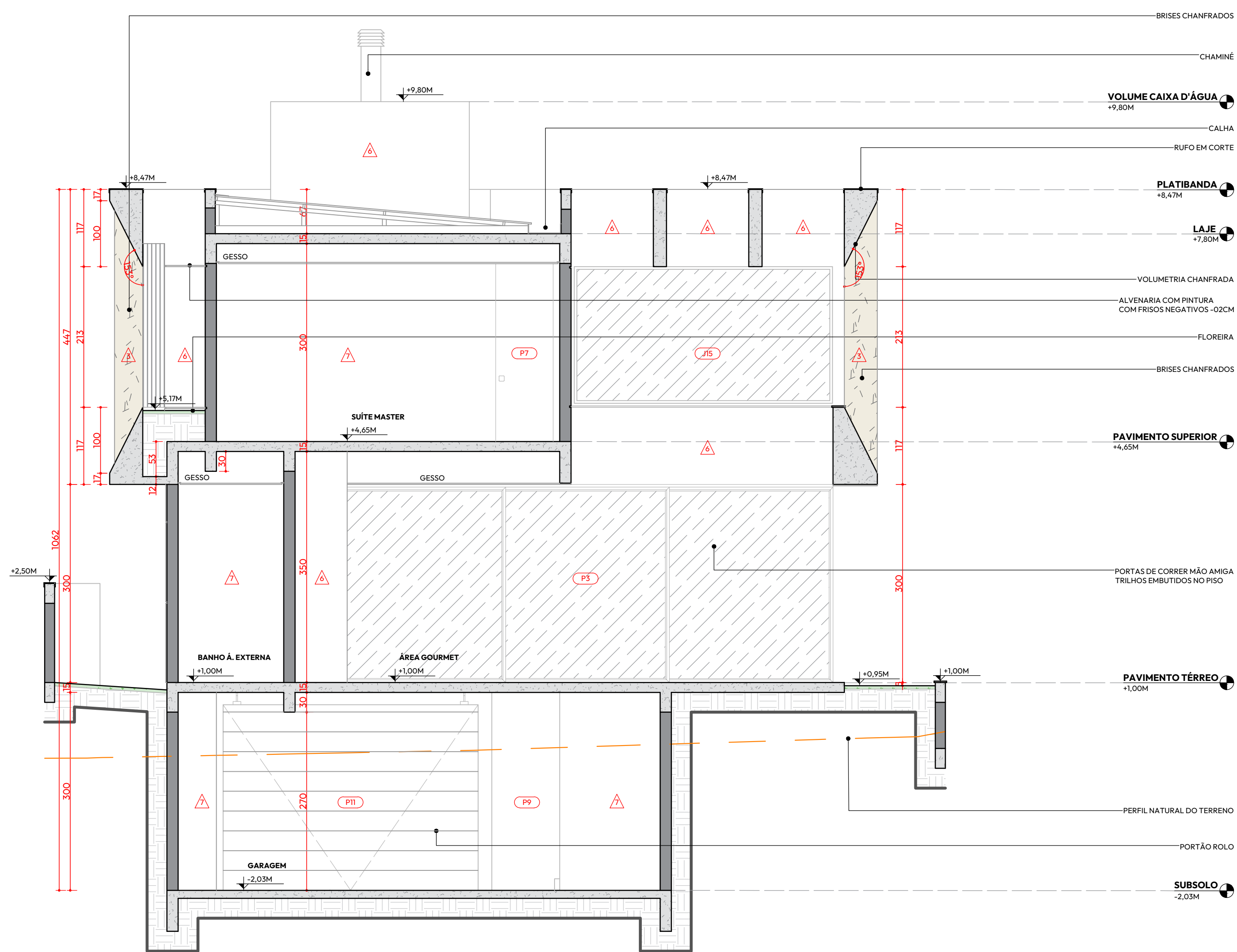
08 CORTE B/B ESCALA: 1/50
