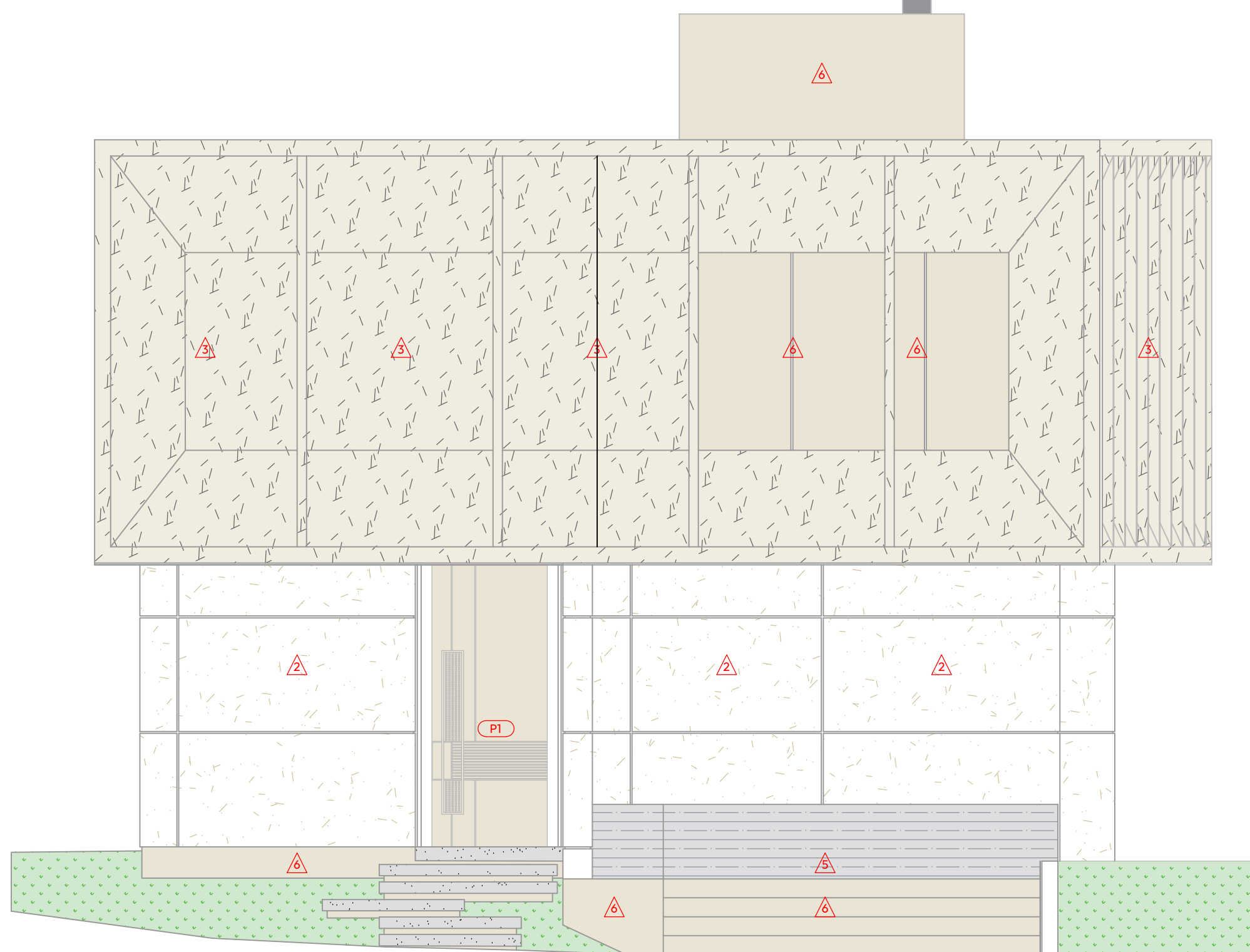
15 FACHADA FRONTAL - E.01 ESCALA: 1/50
