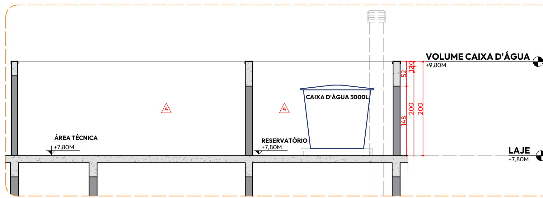
08 CORTE G/G - RESERVATÓRIO ESCALA: 1/50
