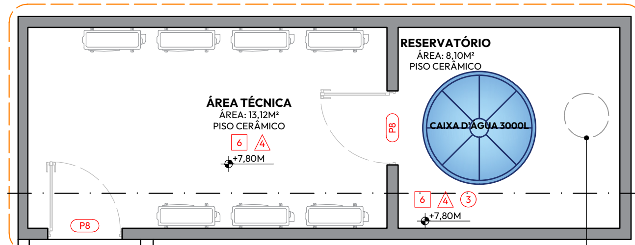
07 PLANTA BAIXA RESERVATÓRIO ESCALA: 1/50
