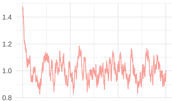
Hierarchical MCMC Trace Plots (Sub
