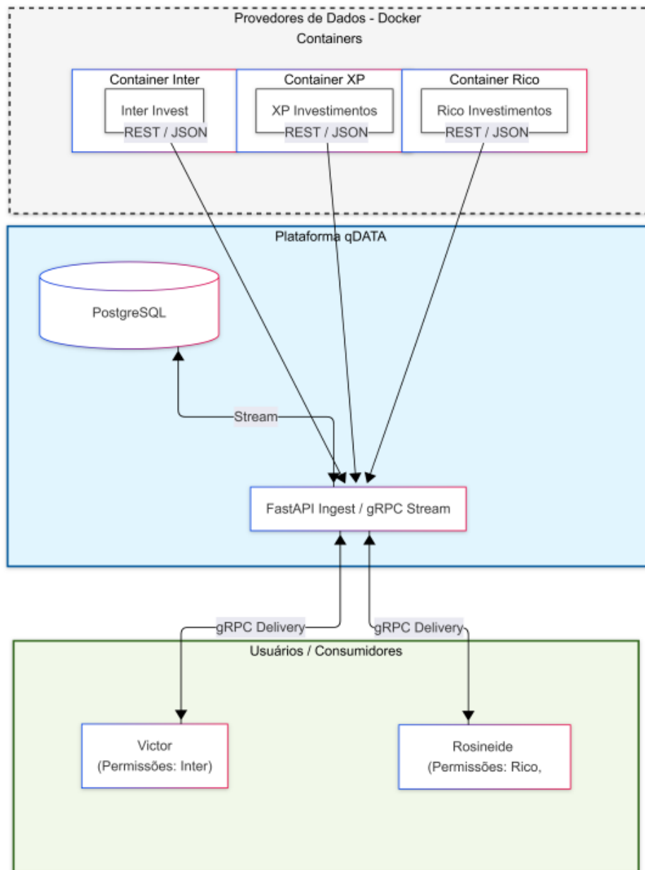
Figura 2 – Visão geral da arquitetura: Ingestão distribuída e distribuição segura de dados financeiros.
