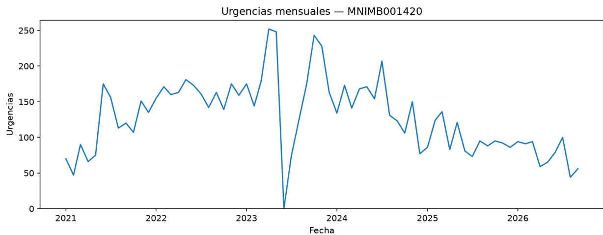
Figura 4: Urgencias mensuales
