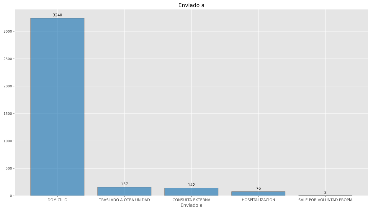
Figura 13: Enviado a
