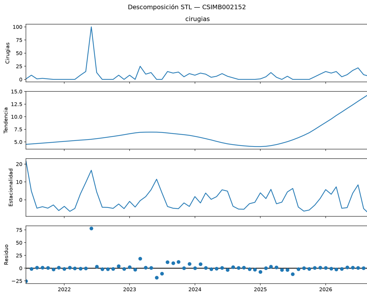
Figura 5: Descomposición STL
